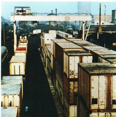
Original DB-Containerkran
